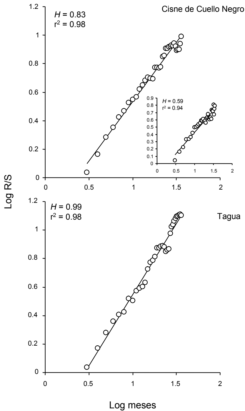
Figura 140. Relación de escalamiento entre el número de meses utilizados para estimar la tasa de cambio poblacional y el rango (R) re-escalado por la desviación estándar (S) para el Cisne de cuello negro y la Tagua para el periodo 1999-2005. La pendiente de la relación corresponde al exponente de Hurst, H .
