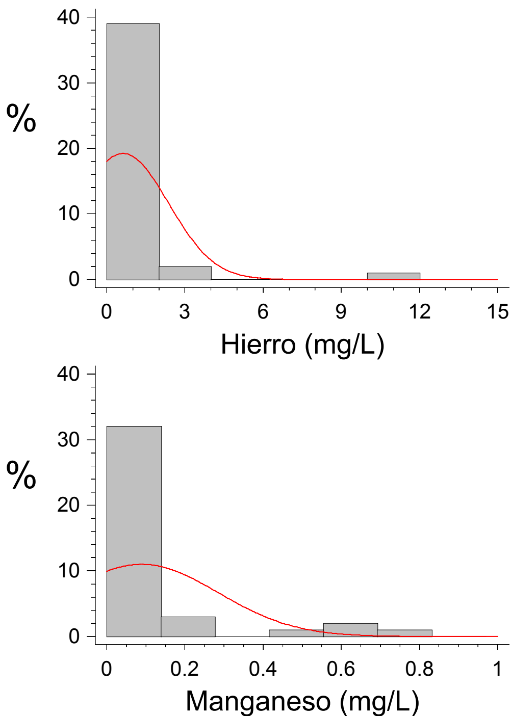
Figura 1. Distribución de frecuencias de las concentraciones de Hierro y Manganeso en aguas subterráneas de Valdivia (fuente de los datos: Tabla 3).
