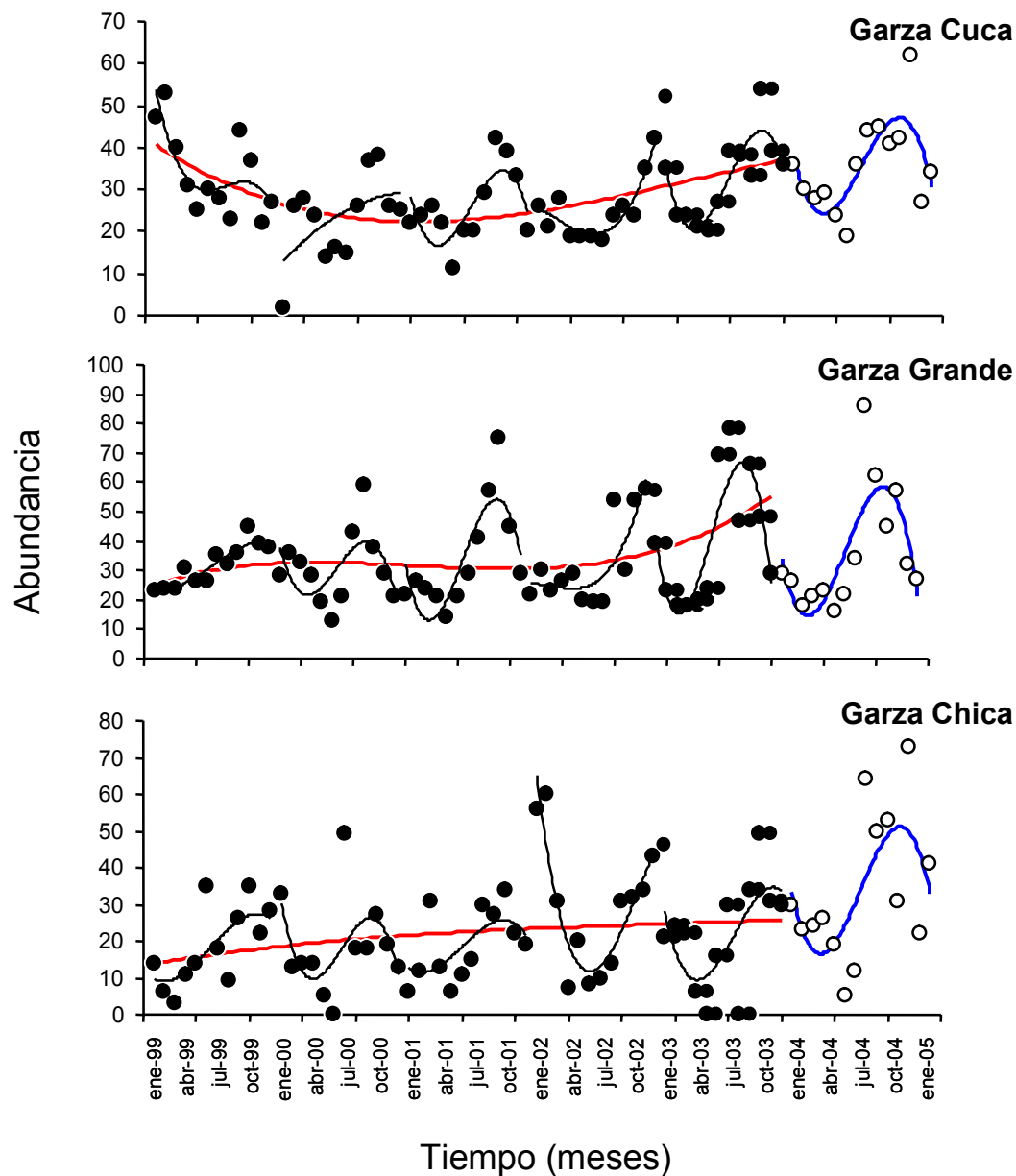
Figura 136. Abundancia poblacional de la Garza Cuca, la Garza Grande y la Garza Chica registrada en el periodo 1999-2005. En todos los casos, la línea roja (puntos negros) muestra la tendencia temporal dominante desde Enero de 1999 a Diciembre del 2003. La línea azul (puntos blancos) representa la tendencia temporal dominante desde Enero del 2004 a Febrero del 2005. Las líneas continuas en color negro representan la tendencia intra-anual para los años 1999, 2000, 2001, 2002 y 2003. La tendencia corresponde a un ajuste polinomial de 3er orden.
