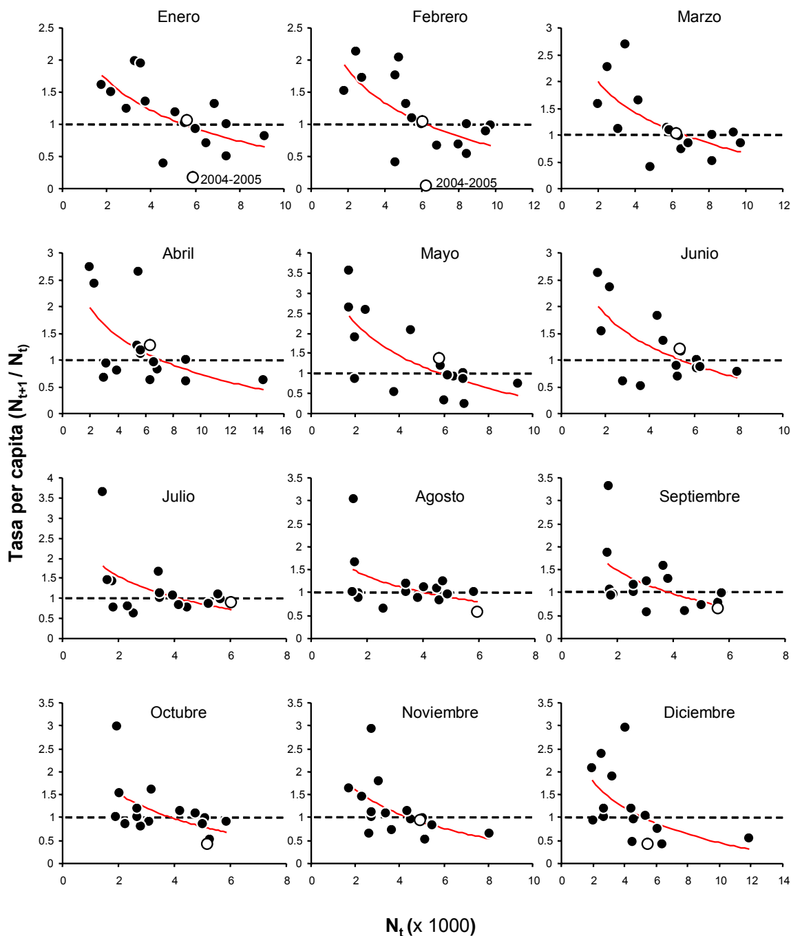
Figura 143. Relación entre la abundancia poblacional y la tasa de cambio anual per capita del Cisne de cuello negro para cada mes del periodo Enero 1988-Febrero 2005. Los círculos blancos indican los valores correspondientes a la tasa de cambio registrada entre el 2003 y el 2004 de cada mes. En los meses de Enero y Febrero se indica la tasa de cambio registrada entre el 2004 y el 2005. La línea continua corresponde a la tendencia descrita mediante el ajuste de un modelo logarítmico. La línea segmentada divide la zona de incrementos (valores positivos) y decrementos (valores negativos) en la tasa per capita de cambio poblacional mensual.
