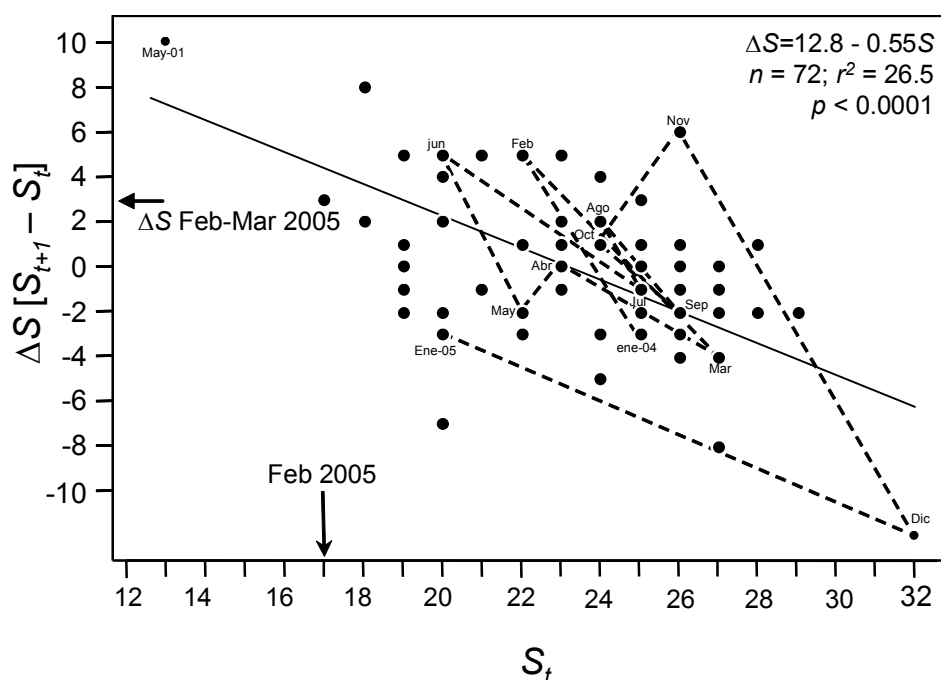
Figura 128. Relación entre la riqueza de especies S en el mes ( t ) y tasa de cambio en el número de especies ( \Delta S ) entre el mes ( t ) y el siguiente ( t+1 ). Los valores positivos y negativos de \Delta S reflejan, respectivamente, incrementos o decrementos en el número de especies. La línea achurada une los datos registrados desde Enero del 2004 hasta Enero del 2005. Se destaca la tasa máxima de incremento registrada en Mayo del 2001. La línea continua corresponde a la línea de regresión estimada por el método de mínimos cuadrados cuyos resultados se muestran en la esquina superior derecha. Las flechas indican el valor de S registrado en Febrero 2005 (17 especies) y la tasa de cambio esperada para Marzo del 2005 (incremento en 3 especies) según este modelo lineal.
