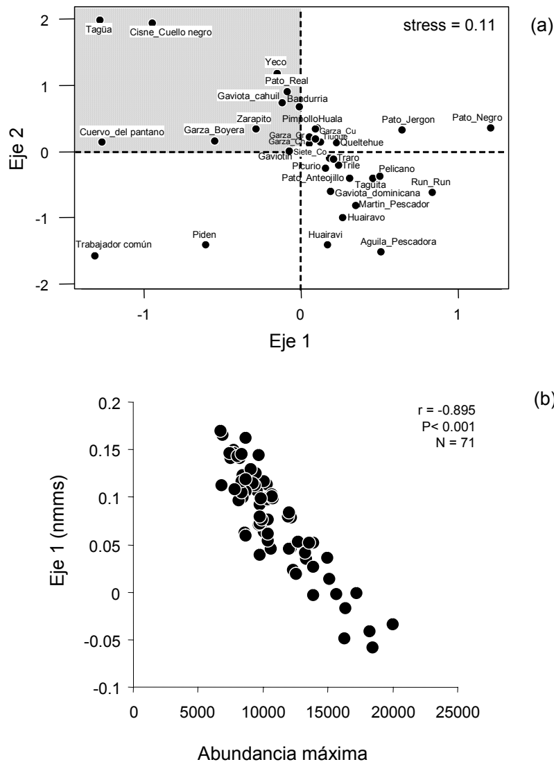
Figura 133. (a) Patrón de ordenación de la avifauna del Santuario descrito por los dos primeros ejes resultantes del análisis de escalamiento no-métrico multidimensional y utilizando la matriz de abundancia poblacional de las 36 especies para el periodo 1999-2005. La zona achurada incluye especies de alta abundancia poblacional y alta variabilidad temporal en la abundancia, (b) relación entre el primer eje de ordenación del ensamble de aves y la abundancia máxima (agrupando a las especies) registrada durante el periodo de estudio. Aunque incluidos en el análisis, no se muestran para claridad los mínimos extremos en abundancia registrados durante Mayo del 2001, Enero y Febrero del 2005.
