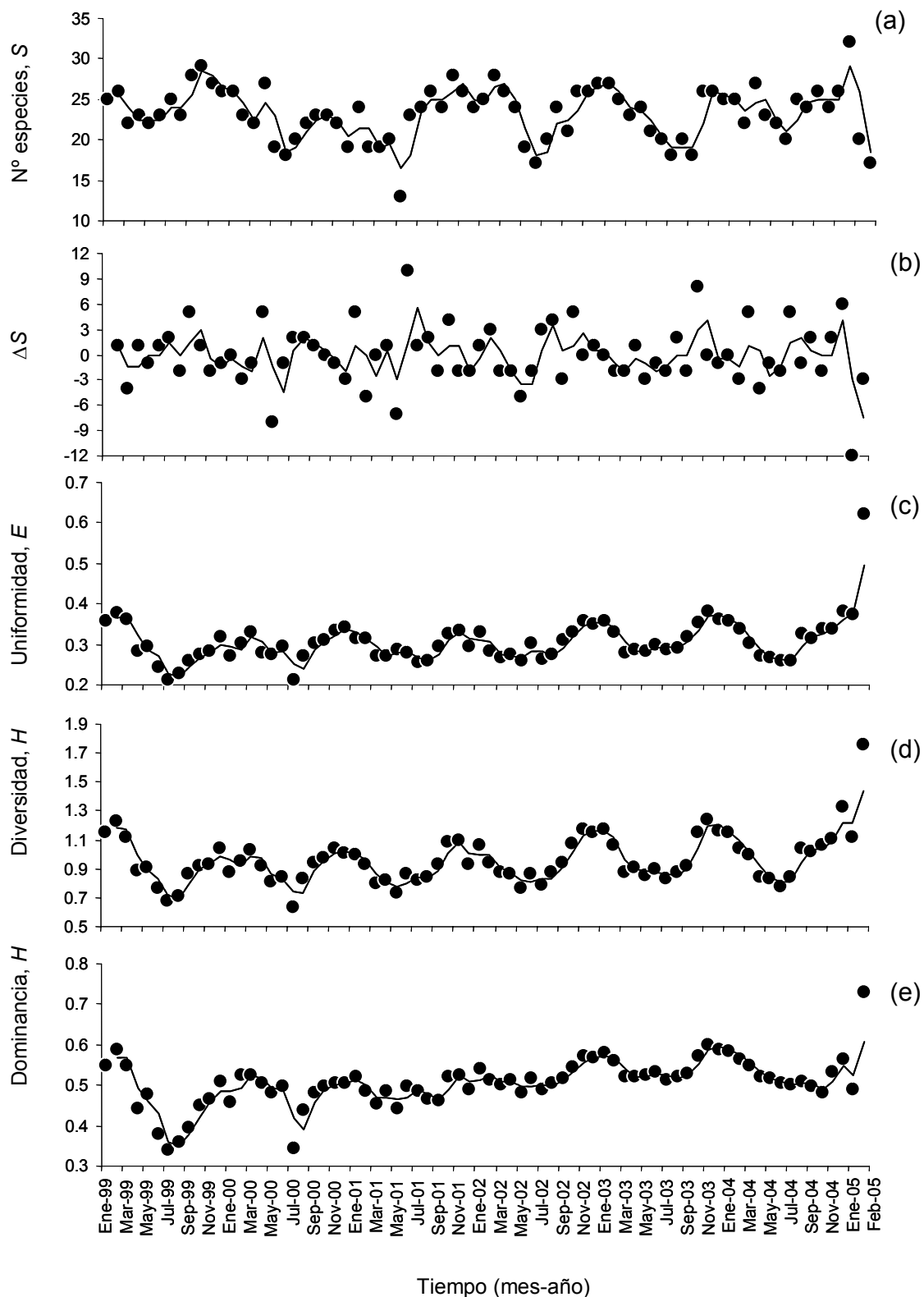
Figura 127. (a) Fluctuaciones en el número de especies de la avifauna del Santuario, (b) tasa de cambio mensual en el número de especies, (c) uniformidad, (d) diversidad de Shannon, (e) dominancia para el ensamble de aves registradas en el Santuario durante el periodo 1999-2005.
