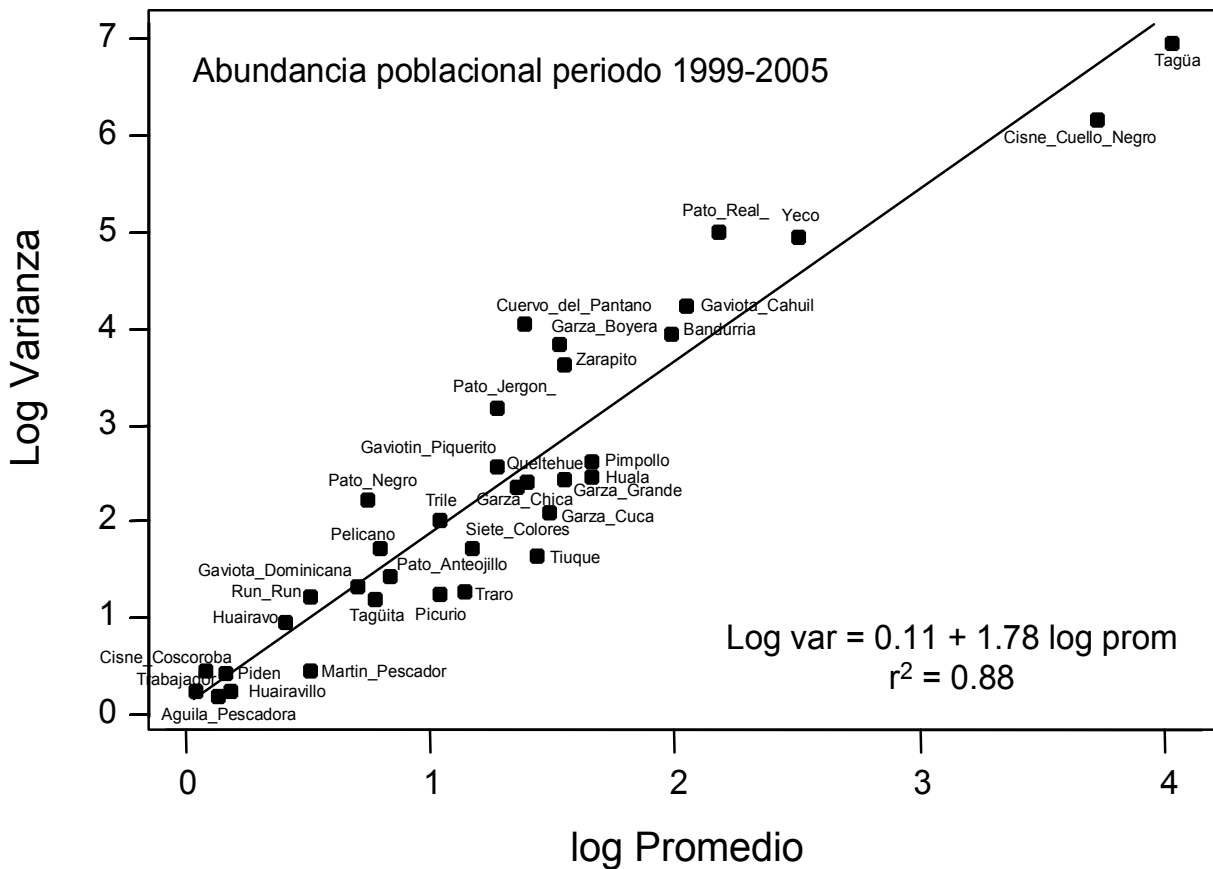
Figura 130. Relación de escalamiento (Ley de Taylor) entre el promedio y la varianza de la abundancia poblacional de todas las especies registradas en el Santuario durante el periodo 1999-2005. La línea corresponde a la predicción de la regresión lineal para los datos logaritmizados.
