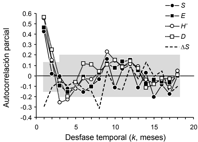
Figura 129. Funciones de autocorrelación para las series de tiempo del número de especies (S), uniformidad (E), diversidad de Shannon ( H' ), dominancia (D) y tasa de cambio en el número de especies ( \Delta S ). La zona achurada corresponde a la zona de aceptación del estadígrafo-t, las correlaciones localizadas fuera de esta zona son significativamente distintas de cero.
