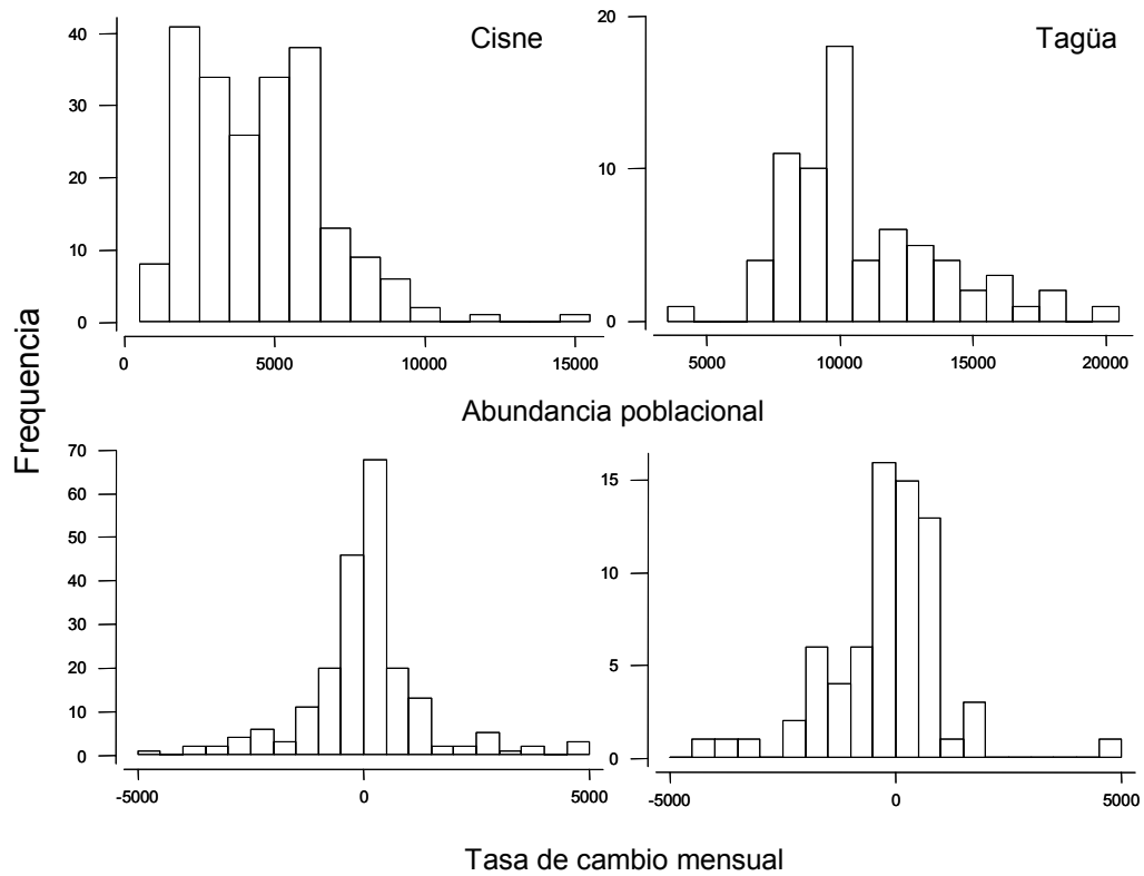
Figura 139. Distribución de frecuencias de la abundancia poblacional y tasa de cambio mensual para el Cisne de cuello negro (periodo 1987-2005) y la Tagua (periodo 1999-2005).
