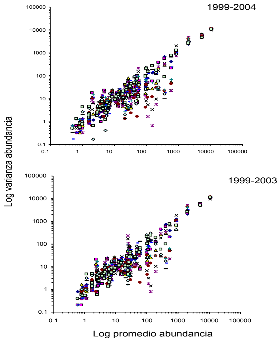
Figura 132. Relación de escalamiento (Ley de Taylor) entre el promedio y la varianza de la abundancia poblacional mensual de una especie ( n=36 ) durante el periodo 1999-2004 (arriba) y para el periodo 1999-2003 (abajo). La línea corresponde a la predicción de la regresión lineal de los datos logaritmizados.
