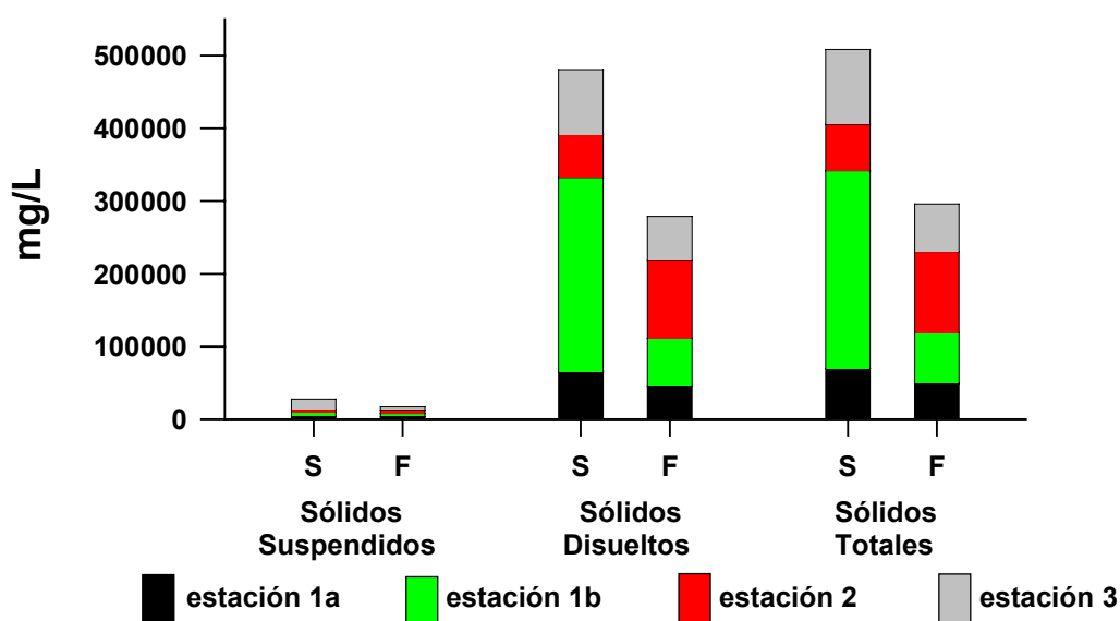
Figura 22. Cargas netas diarias de Sólidos Suspendedos, Disueltos y Totales (Suspendedos + Disueltos) en las aguas de superficie y fondo de las cuatro estaciones de muestreo en el río Cruces.
