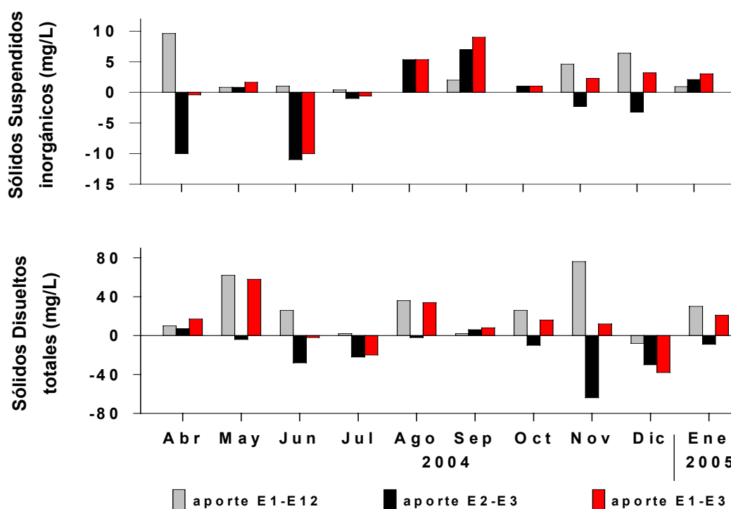
Figura 50. Aporte en la concentración de Sólidos Suspendedos inorgánicos y Sólidos Disueltos totales entre las estaciones 1y 2 (aporte E1-E2), 2 y 3 (aporte E2-E3) y entre las estaciones 1 y 3 (aporte E1-E3) en el río Cruces.
