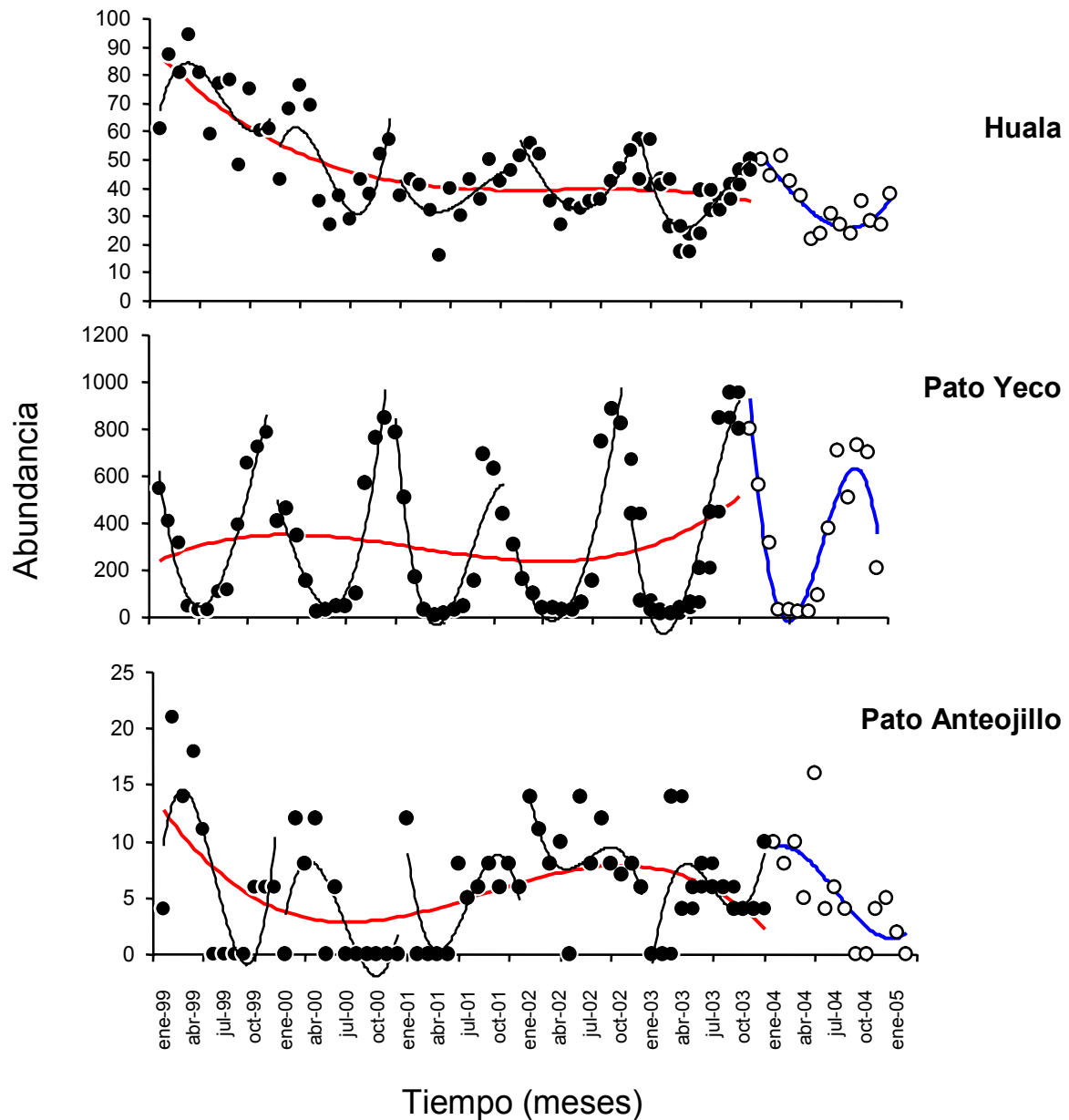
Figura 135. Abundancia poblacional de la Huala, el Pato Yeco y el Pato Anteojillo registrada en el periodo 1999-2005. En todos los casos, la línea roja (puntos negros) muestra la tendencia temporal dominante desde Enero de 1999 a Diciembre del 2003. La línea azul (puntos blancos) representa la tendencia temporal dominante desde Enero del 2004 a Febrero del 2005. Las líneas continuas en color negro representan la tendencia intra-anual para los años 1999, 2000, 2001, 2002 y 2003. La tendencia corresponde a un ajuste polinomial de 3er orden.
