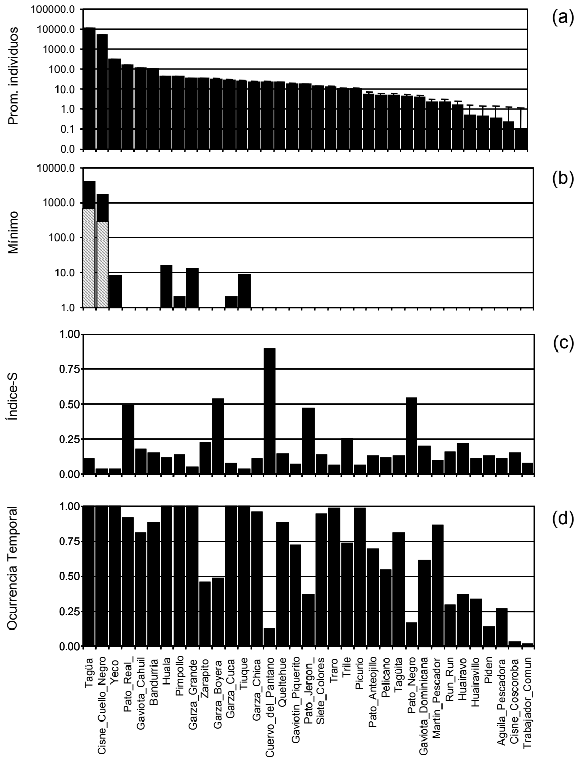
Figura 125. (a) Promedio de individuos ( \pm 1 D.E.) registrados durante el periodo 1999-2005 para la avifauna del Santuario, (b) abundancia mínima de individuos registrada para el periodo 1999-2004 (barras negras) y para Enero y Febrero del 2005 (barras achuradas), (c) variabilidad temporal de la abundancia individual de la avifauna caracterizada por el índice-S, (d) ocurrencia temporal de cada especie expresada como la razón entre el número de muestreos en que una determinada especie estuvo presente y el total de muestreos.
