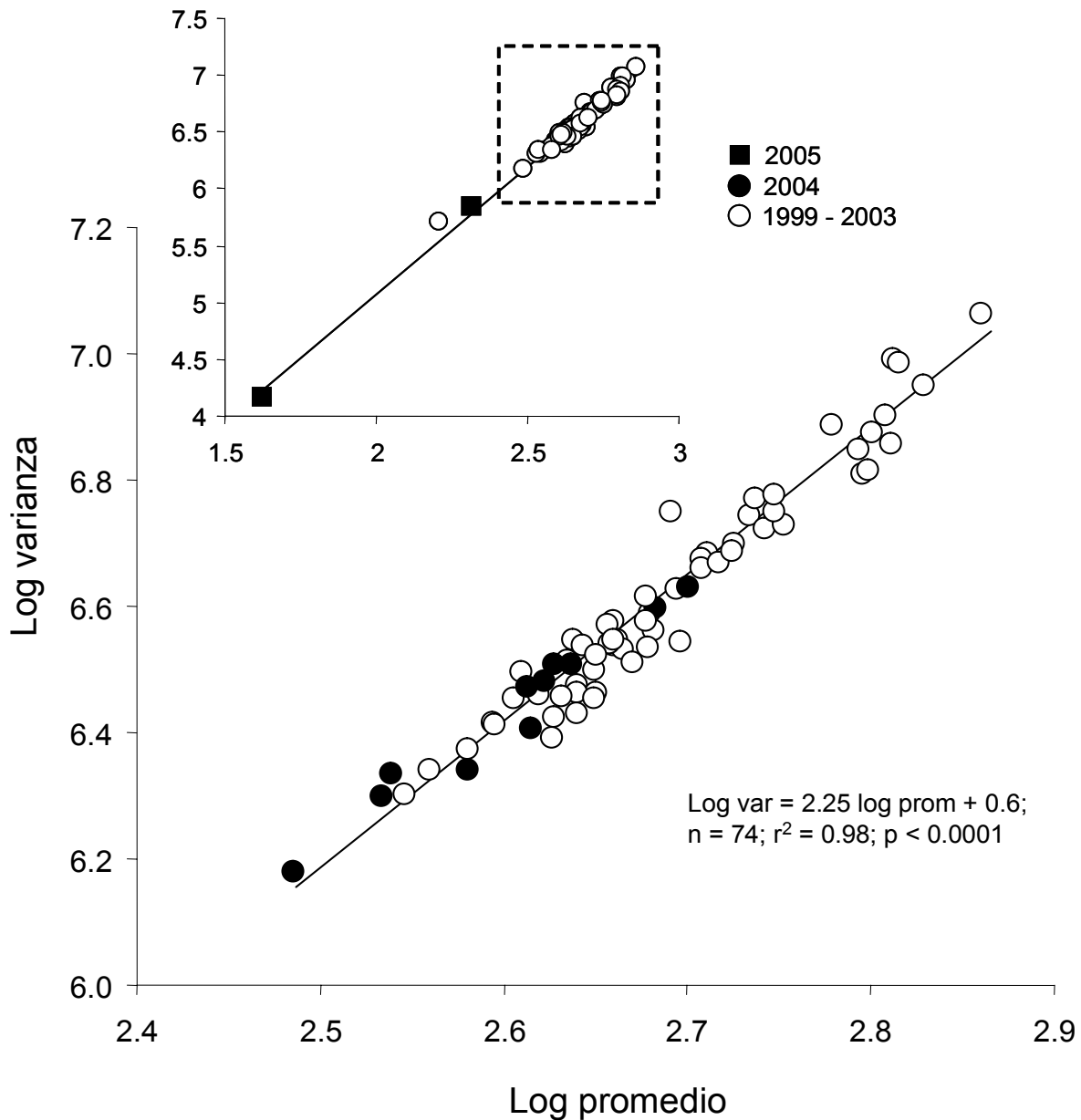
Figura 131. Relación de escalamiento (Ley de Taylor) entre el promedio y la varianza de la abundancia de individuos (agrupando todas las especies de aves) registrada en el Santuario durante el periodo 1999-2005 (arriba inserto). Abajo se muestra la relación ampliada para el periodo 1999-2004. La línea corresponde a la predicción de la regresión lineal de los datos logaritmizados.
