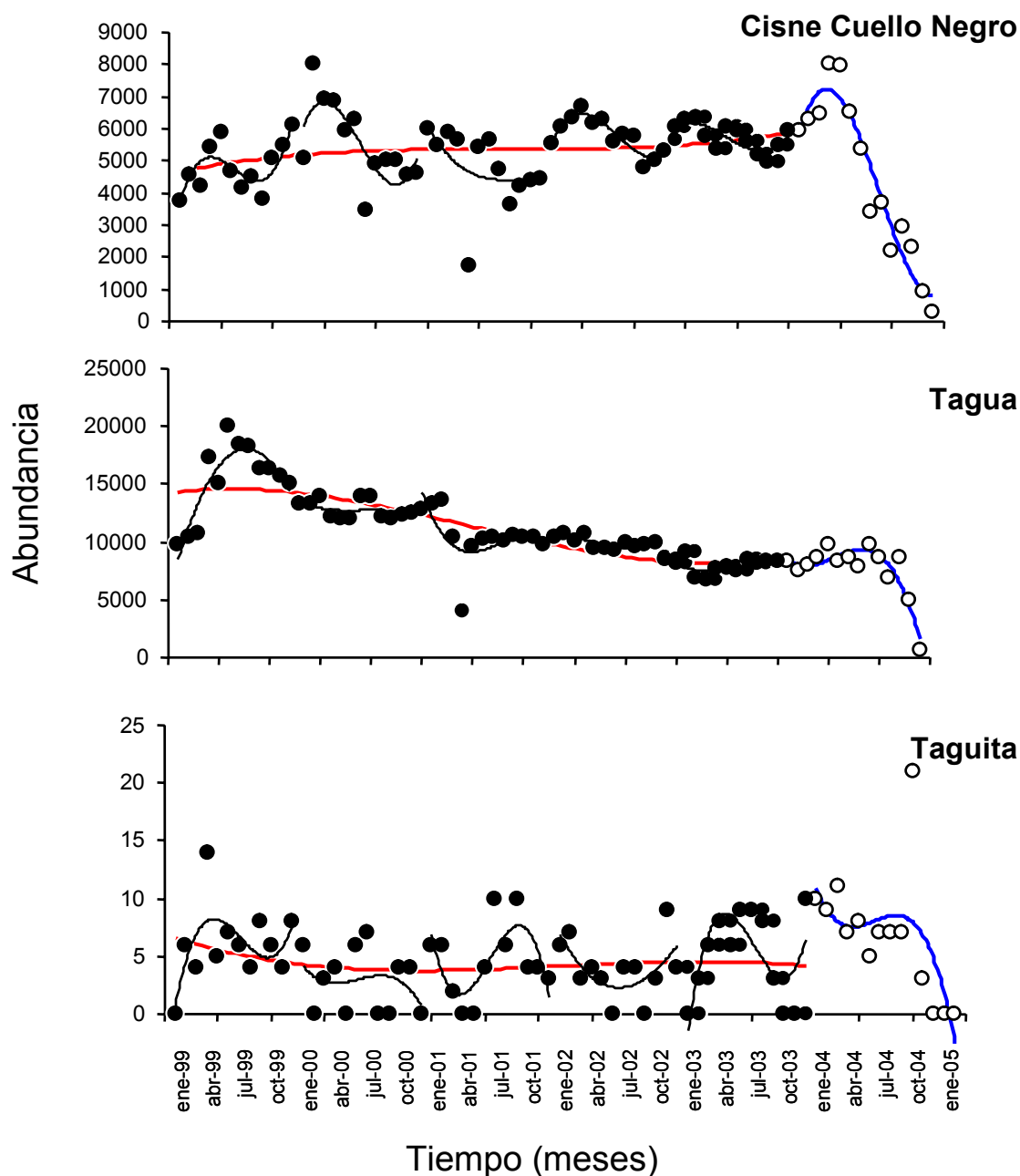
Figura 134. Abundancia poblacional del Cisne de cuello negro, la Tagua y la Taguita durante el periodo 1999-2005. En todos los casos, la línea roja (puntos negros) muestra la tendencia temporal dominante desde Enero de 1999 a Diciembre del 2003. La línea azul (puntos blancos) representa la tendencia temporal dominante desde Enero del 2004 a Febrero del 2005. Las líneas continuas en color negro representan la tendencia intra-anual para los años 1999, 2000, 2001, 2002 y 2003. La tendencia corresponde a un ajuste polinomial de 3er orden.
