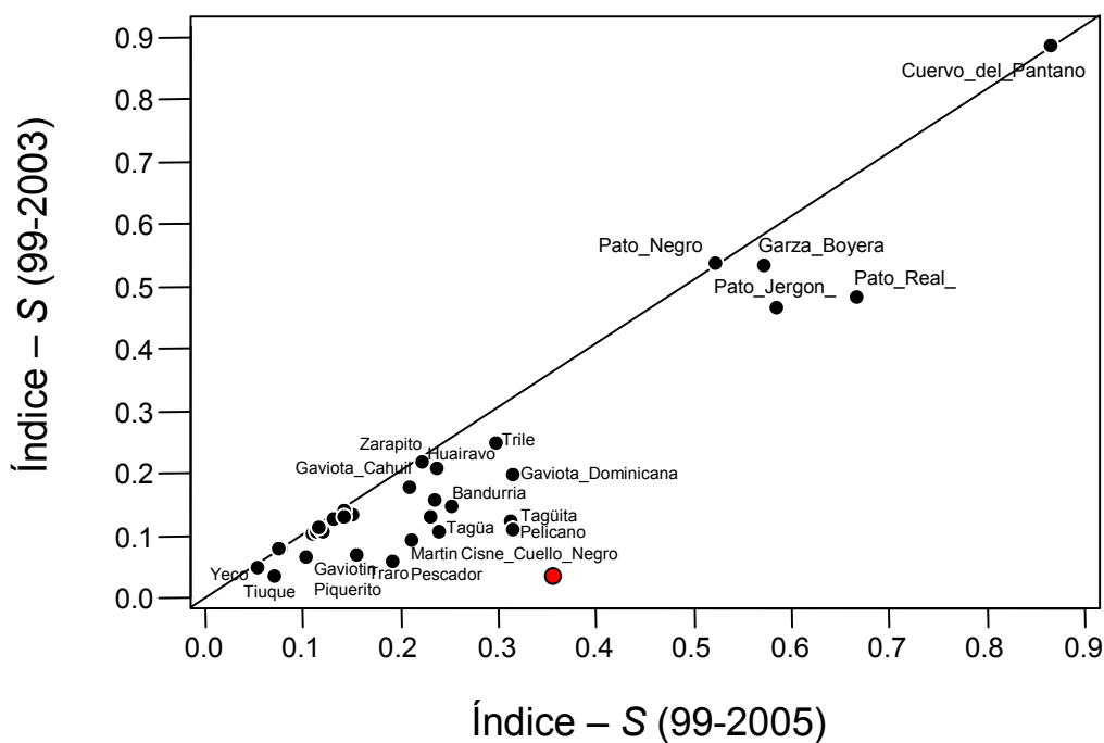
Figura 126. Relación entre la variabilidad temporal de las fluctuaciones en abundancia de cada especie registrada durante el periodo 1999-2005 y la variabilidad temporal registrada durante 1999-2004. La bisectriz indica una relación 1:1 en la variabilidad temporal para ambos periodos de estudios. En rojo se identifica la relación para el Cisne de cuello negro.
