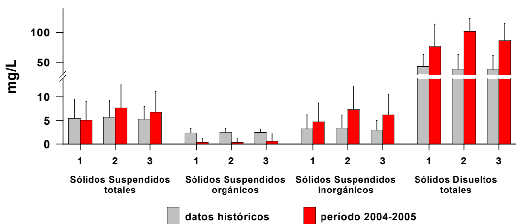
Figura 78. Valores de promedios históricos y actuales (período 2004-2005) de las concentraciones de Sólidos Suspendedos (totales, orgánicos e inorgánicos) y Sólidos Disueltos totales en las aguas de las tres estaciones analizadas en el río Cruces..
