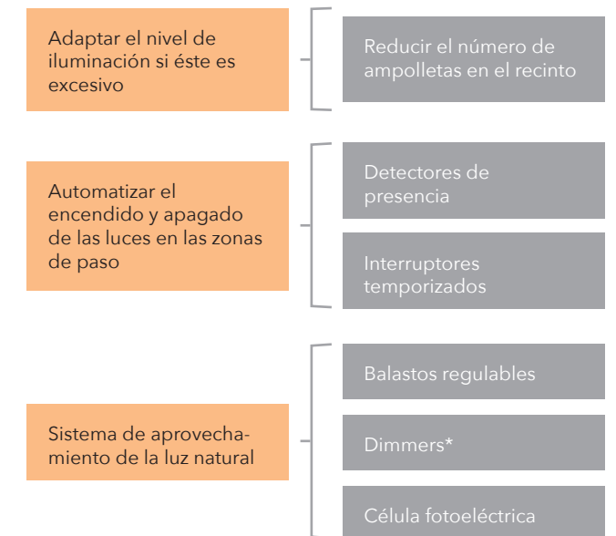
Figura 8. Medidas de Mejora de Eficiencia Energética en iluminación: medidas de gestión.
