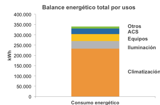
Gráfico 6. Ejemplo de balance energético total por usos.
